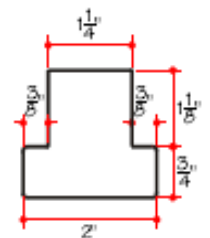
L16 T-POST
