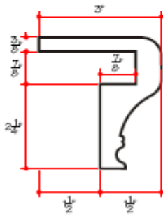
SILL CAP
