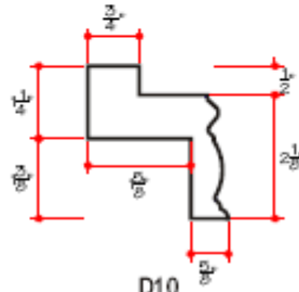
D10 Z-FRAME
